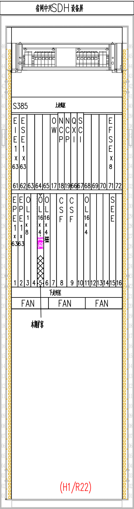
省网A2平面SDH设备机架图
